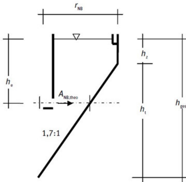
Fig. 80: Hopper Tank, A226
