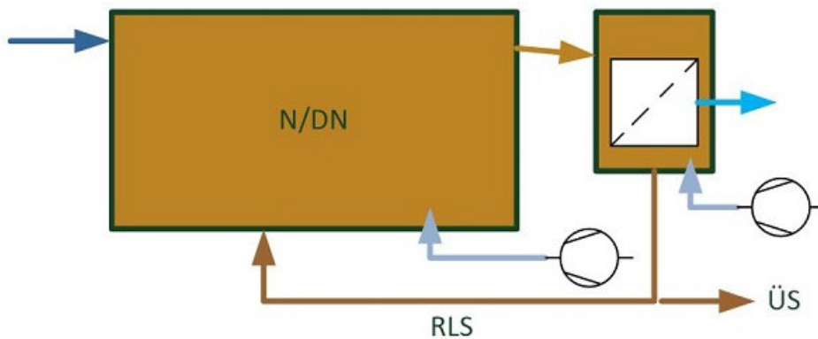
Fig. 112: Intermittend/simultaneous denitrifikation
