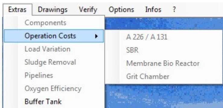
Fig. 141: Menu > Extras
